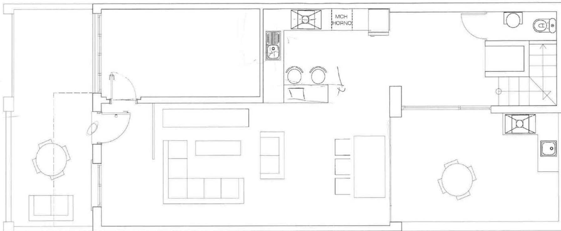
Plano planta baja
