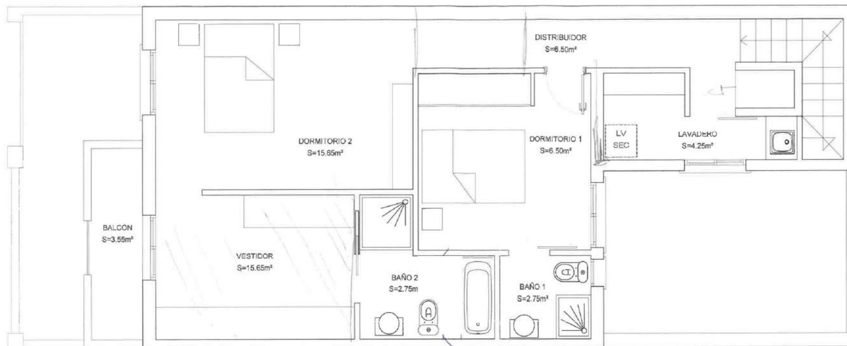
Plano primera planta
